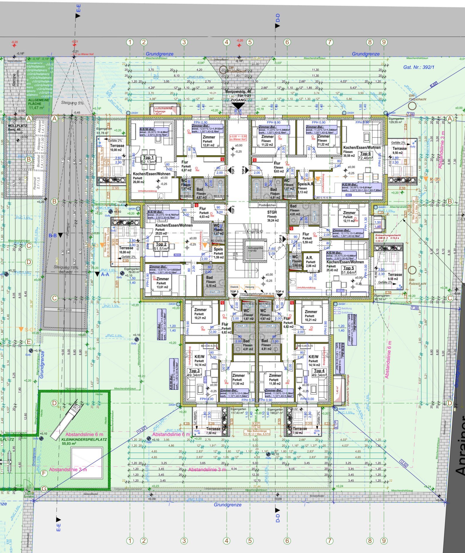
GRUNDRISS ERDGESCHOSS
